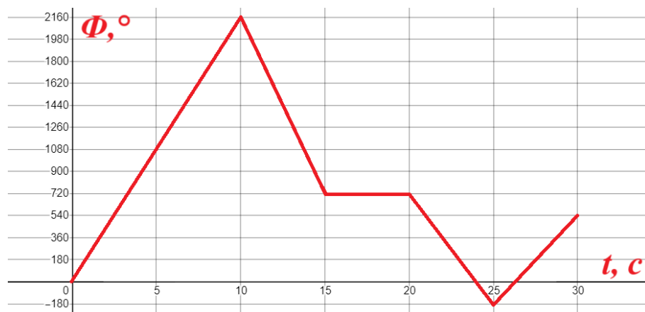
График энкодера мотора
