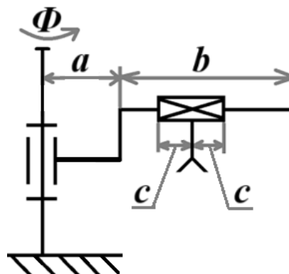
Схема манипулятора
