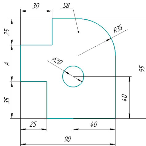
Чертёж
