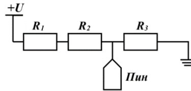
Схема цепи
