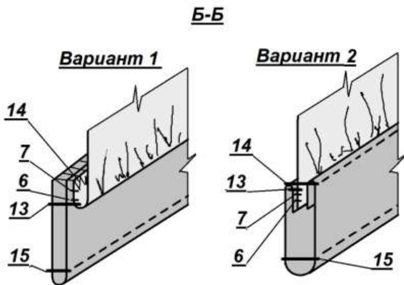
Рисунок 2 – Схемы обработки швов и узлов рукава
