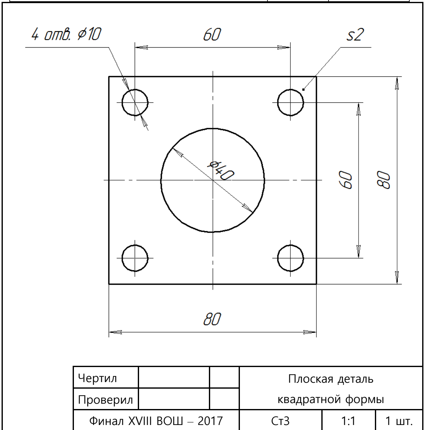
Рис. 1. Образец чертежа плоской детали квадратной формы
